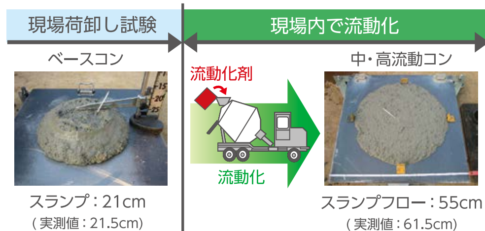
中・高流動コンクリートの製造方法
