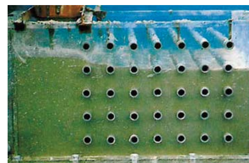
充填性試験(優れた自己充填性)
